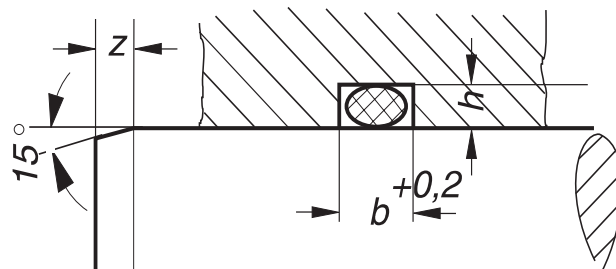
fig.10. Tolerancias de alojamientos
