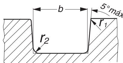
fig.13. Alojamiento rectangular, radios de acabados
