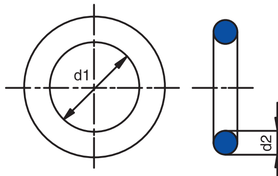
fig.1. Medidas de la Junta Tórica.
