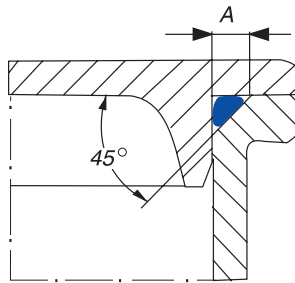
fig.11. Alojamiento triangular.
