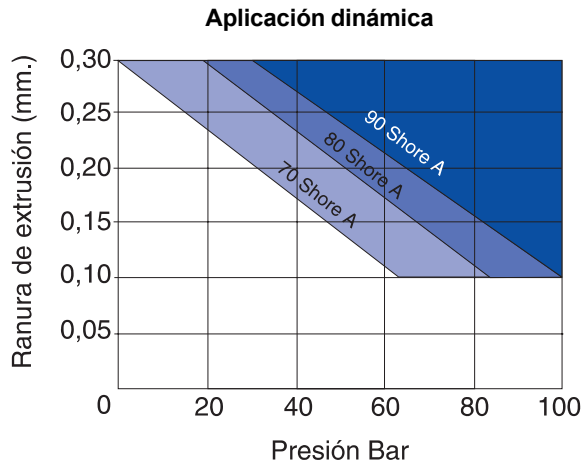
fig.5. Selección de la ranura de extrusión. Aplicación dinámica
