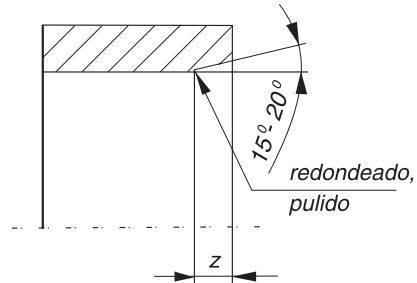
fig.14. Bisel de entrada para cilindros.
