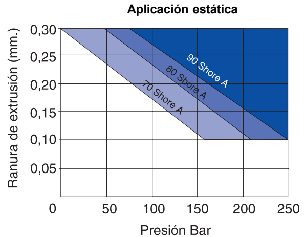
fig.6. Selección de la ranura de extrusión. Aplicación estática.
