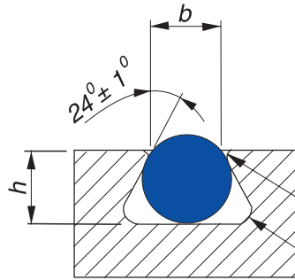
fig.12. Alojamiento trapezoidal.
