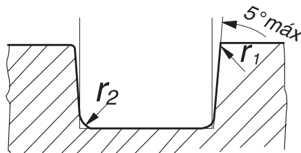
fig. 7. Alojamiento rectangular
