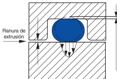
fig.4. Deformación inicial.
