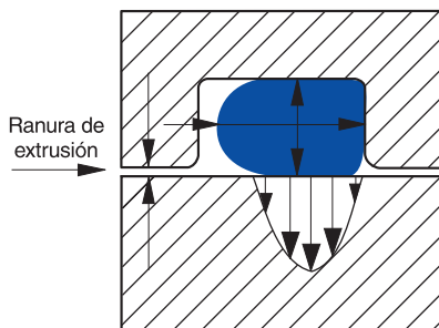
fig.4a. Deformación inicial más presión del sistema.
