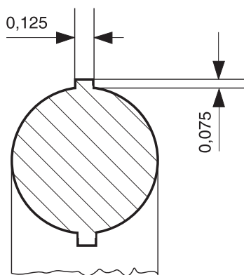
fig.2. Límites máximos de rebabas según ASTM.
