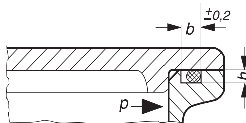
fig. 9. Sellado axial
