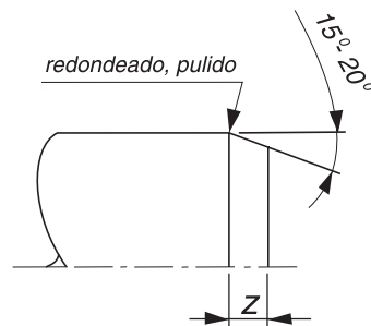
fig.15. Bisel de entrada para vástagos.
