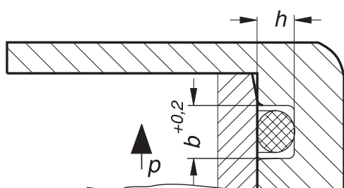
fig. 8. Sellado radial
